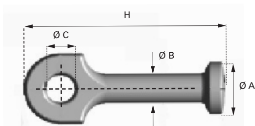
Chiodo O a occhio - Ancre à oeil O
