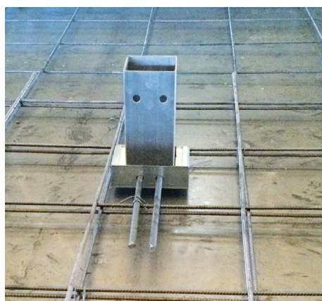
Fondo cassero Fond de coffrage
