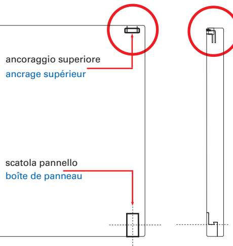
Panneau design - détail
