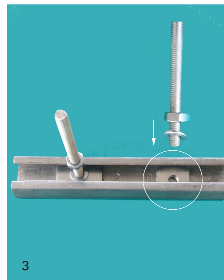
R7 installata - R10 avvitare R7 installé - R10 visser
