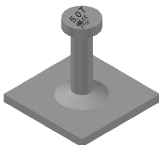
Chiodo P Ancre à semelle
