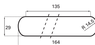
Dettaglio del supporto per piastra PICC2C Détail du support PICC2C
