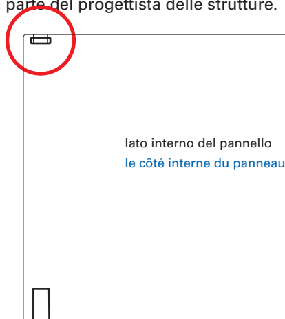
Disegno del pannello - dettaglio
