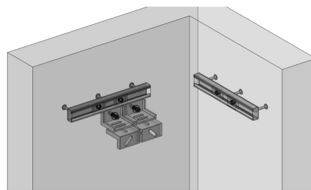
Высокоэффективные смарт-анкеры HGP для сдвигов и динамических нагрузок
