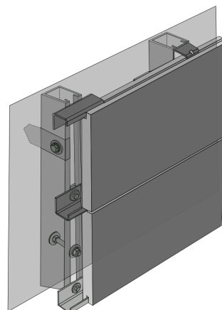
Опоры для вентилируемых фасадов монолитных плит (стандарт CE)
