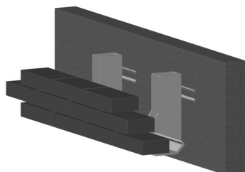
Кронштейны для вентилируемых кирпичных фасадов
