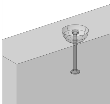
Высокоэффективный подъемный анкер (стандарт CE)
