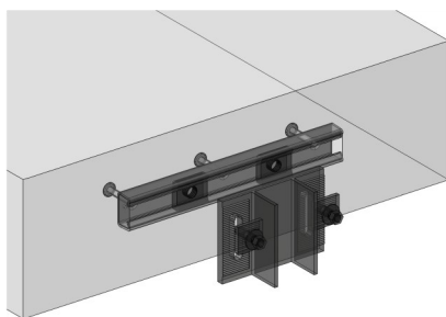
Высокоэффективные смарт-анкеры HGP для сдвигов и динамических нагрузок
