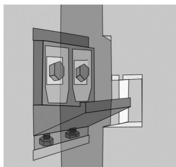
ASP кронштейн для фиксации монолитных панелей
