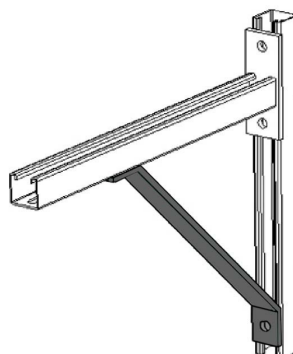
Крепление СОФ и фиксация рельс (СОФ – стационарное оборудование фасадов)
