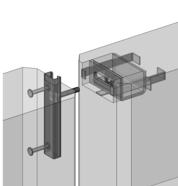
Фиксатор монолитных панелей
