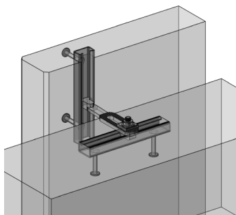
GP анкерная шина (стандарт EC)
