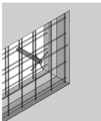
Соединитель для сэндвич -панелей "Link-Loc"
