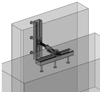
Сейсмостойкая анкерная шина
