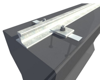
Крепление СОФ и фиксация рельс (СОФ – стационарное оборудование фасадов)
