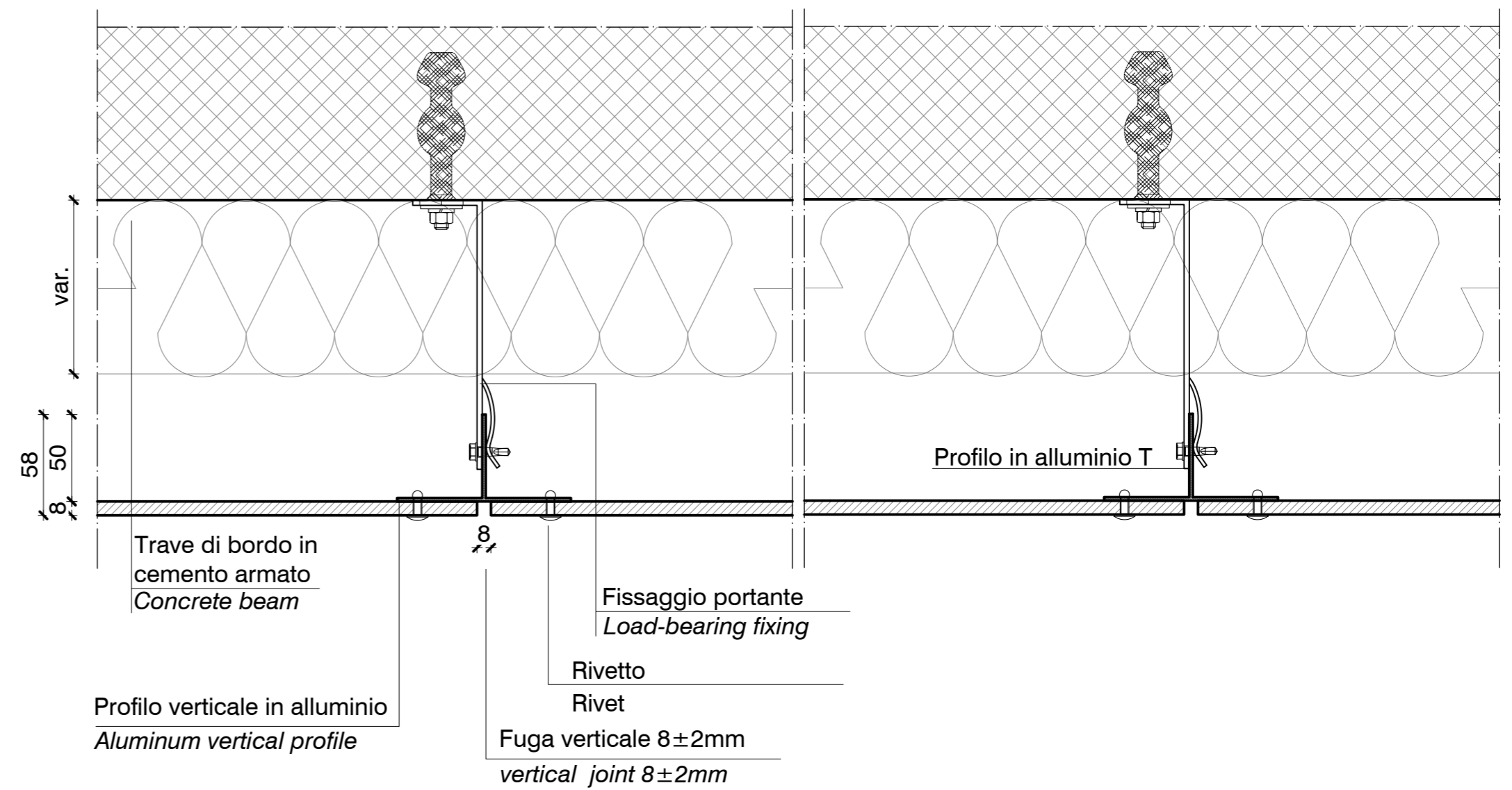
Piastre portanti di fissaggio Load bearing Fixing brackets
