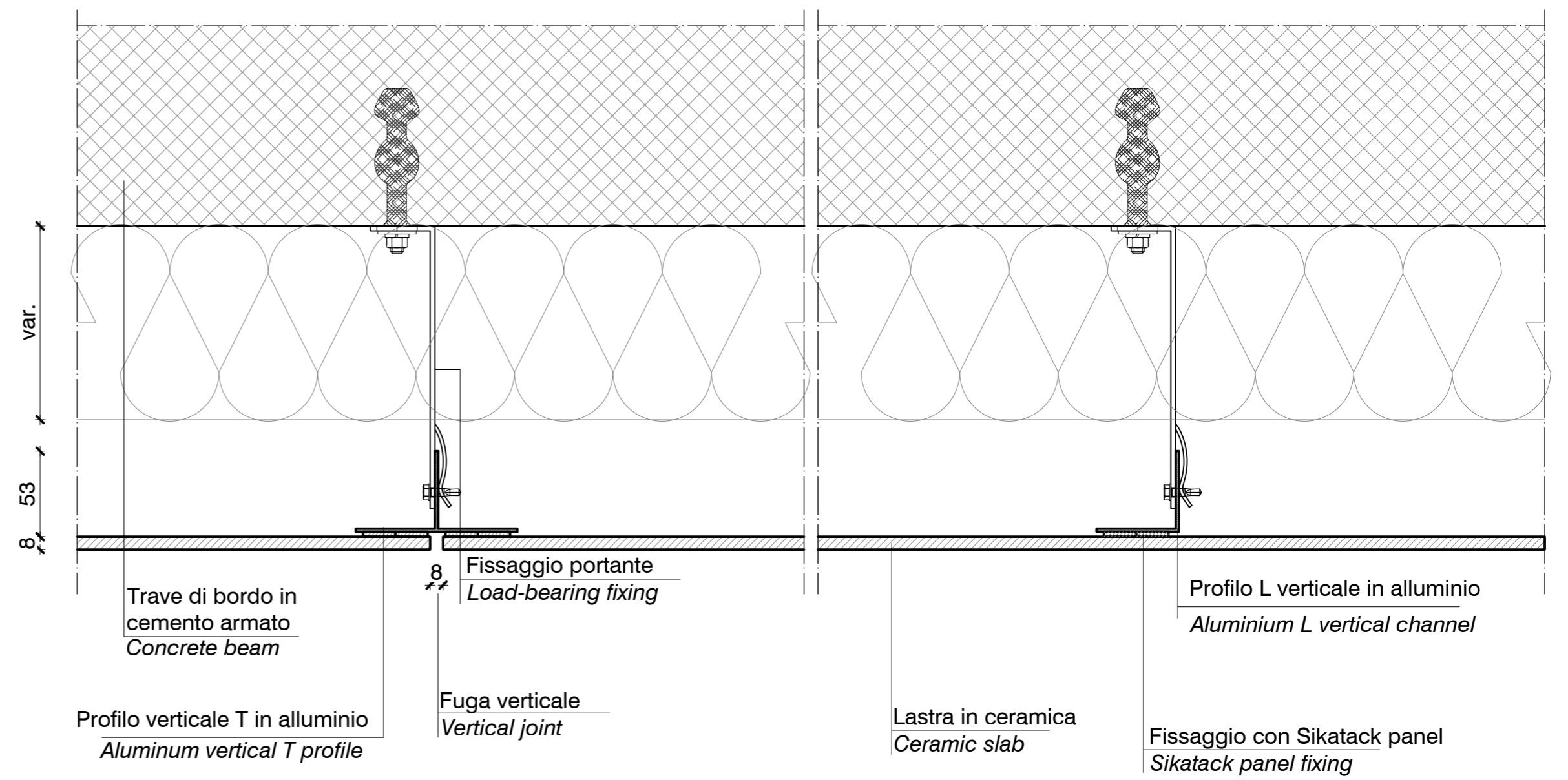
Plastre portanti di fissaggio Load bearing Fixing brackets
