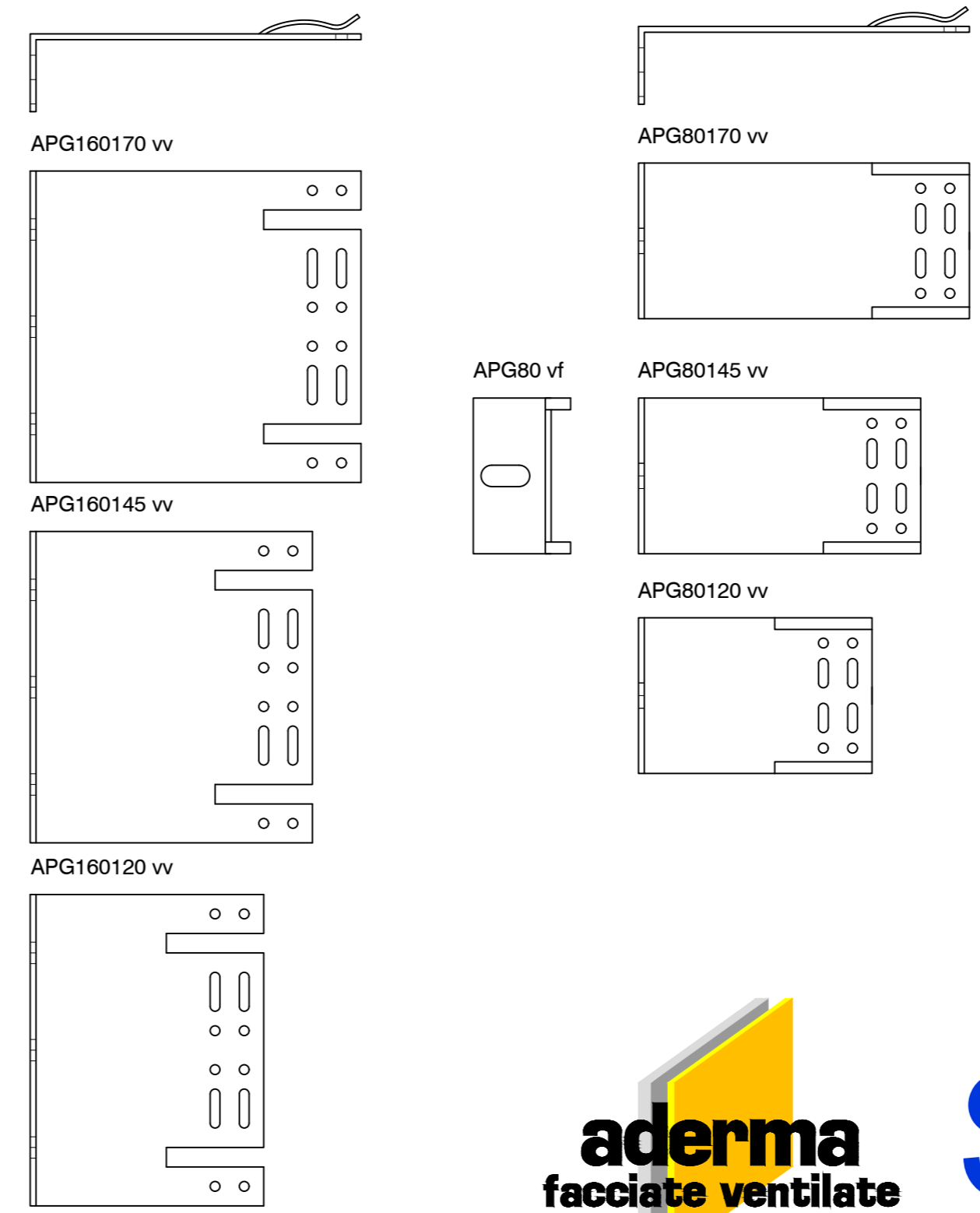
Plastre portanti di fissaggio Load bearing Fixing brackets
